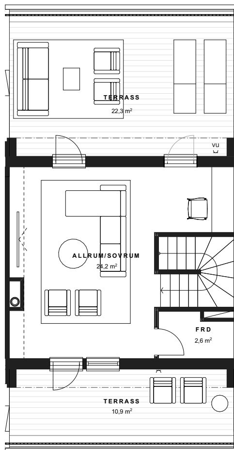
TAKTERRASS
