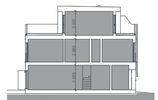
SEKTION
